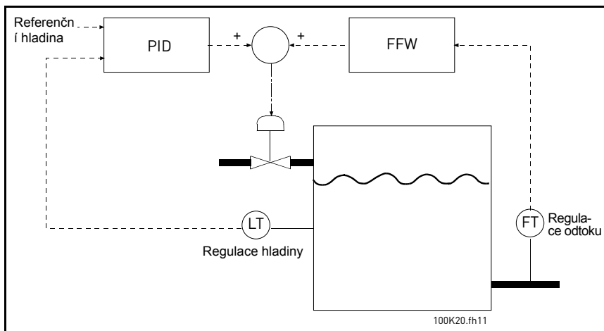
Obr. 34. Dopředná regulace řízení
