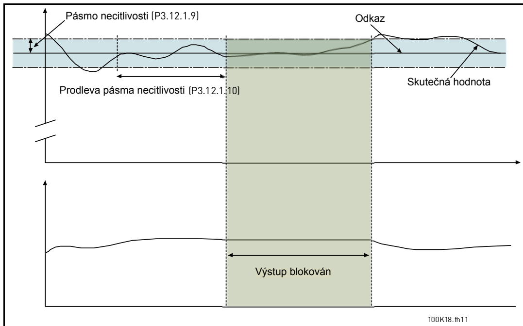
Obr. 32. Pásmo necitlivosti
