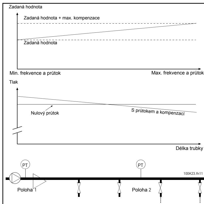
Obr. 37. Povolení kompenzace ztráty tlaku reference 1
