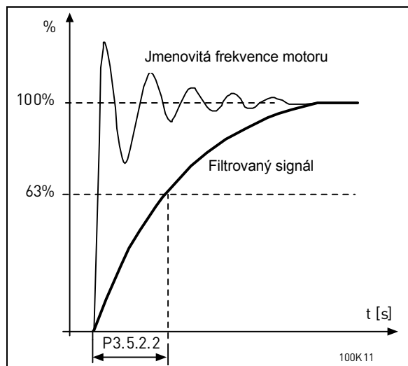
Obr. 24. Filtrování signálu AI1
