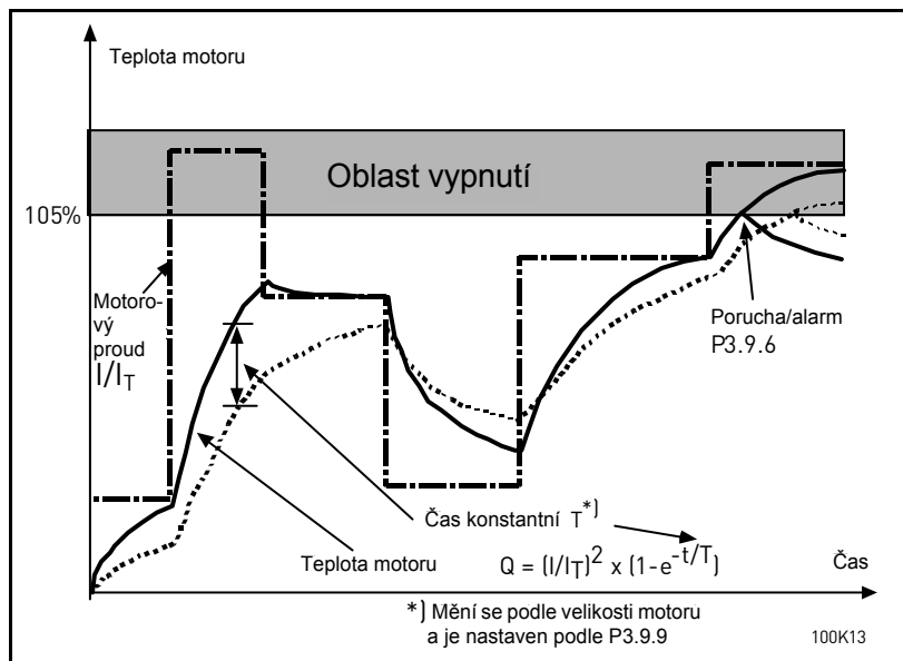
Obr. 26. Výpočet teploty motoru
