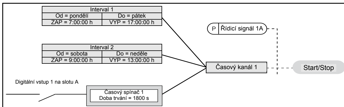
Obr. 16. Konečná konfigurace, ve které je jako řídicí signál pro příkaz start místo digitálního vstupu použit časový kanál 1.
