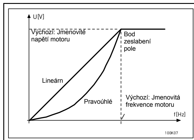
Obr. 17. Lineární a kvadratická změna napětí motoru
