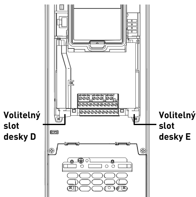
Obr. 13. Sloty doplňkových desek
