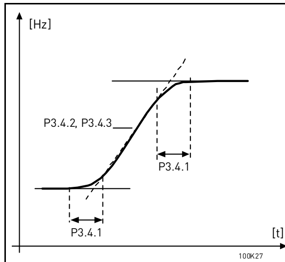
Obr. 23. Rozběh/Doběh (tvar křivky S)
