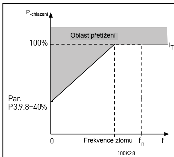
Obr. 25. Křivka proudu I_T při teplotě motoru
