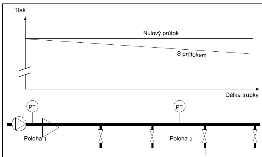
Obr. 36. Umístění snímače tlaku
