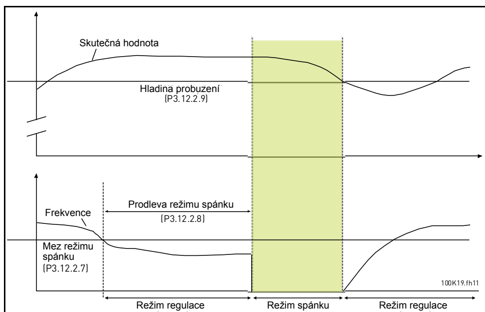
Obr. 33. Klidový limit, Zpoždění klidového režimu, Úroveň restartu
