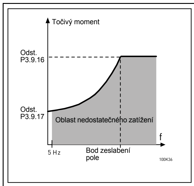
Obr. 29. Nastavení minimálního zatížení
