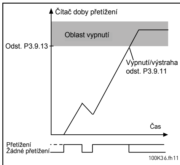
Obr. 28. Čítač času zastavení při přetížení
