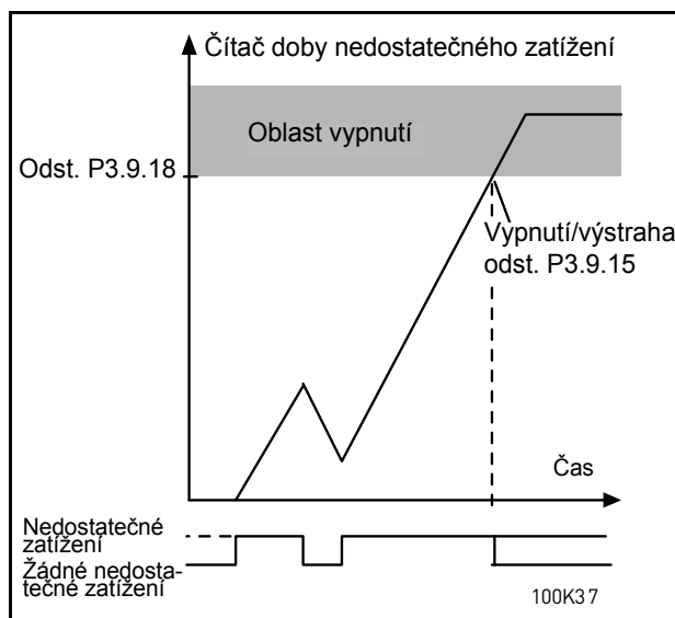
Obr. 30. Funkce čítače doby při podproudu
