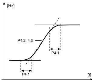
obr. 9.3: Rozběh a doběh ve tvaru S
