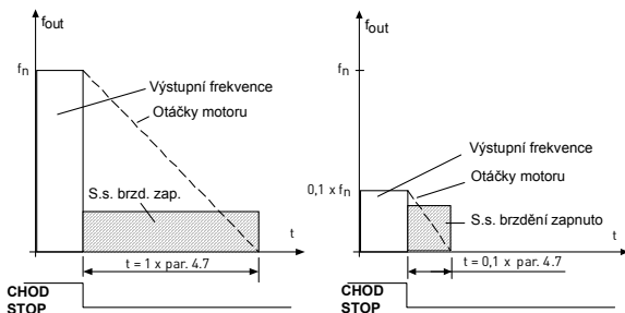
obr. 9.5: Doba s.s. brzdění je-li funkce zastavování = Volný doběh
