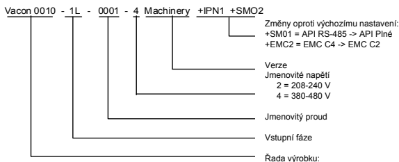
obr. 2.1: Kód označení typu Vacon 10
