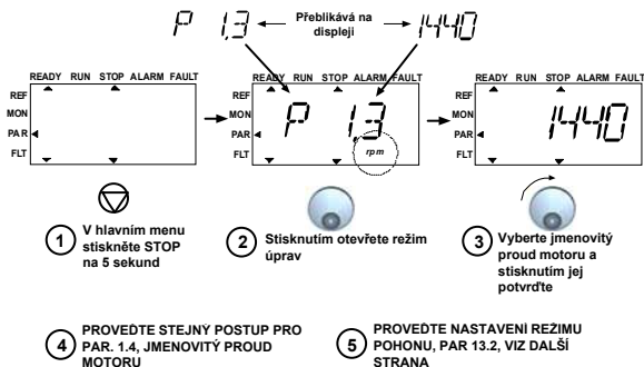
obr. 9.12: Průvodce spuštěním
