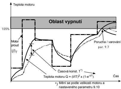
obr. 9.9: Výpočet teploty motoru
