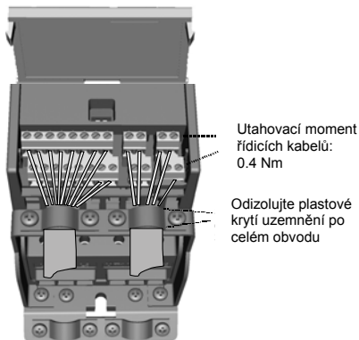
obr. 3.8: Připevněte řídicí kabely. Viz kapitolu 6.1
