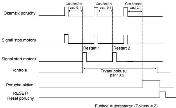
obr. 9.10: Automat. restart
