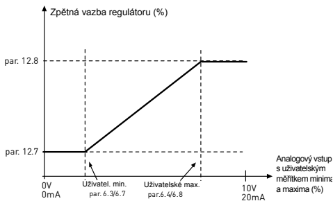
obr. 9.11: Minimum a maximum zpětné vazby
