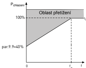
obr. 9.8: Výkon chlazení motoru
