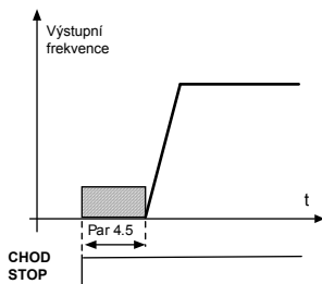
obr. 9.4: Čas s. s. brzdění při spouštění
