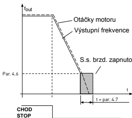
obr. 9.6: Doba s.s. brzdění je-li funkce zastavování = Rampa
