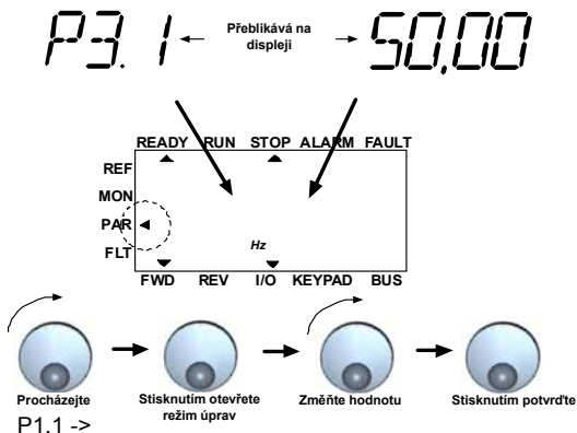
obr. 7.5: Menu Parametr
