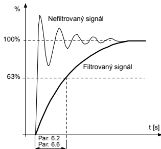
obr. 9.7: Filtrování signálů AI1 a AI2
